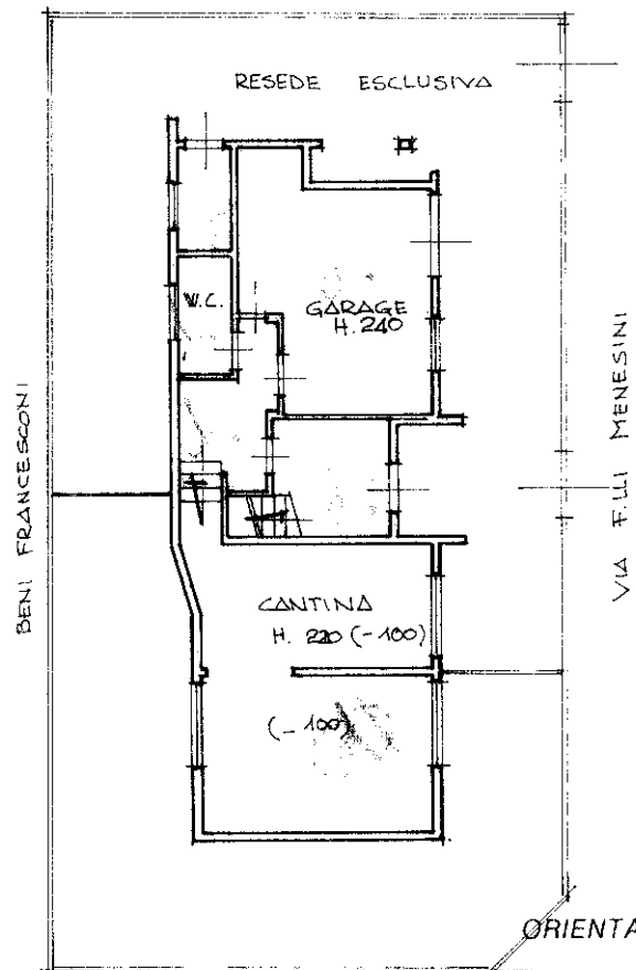
PIANO TERRA E SEMITERRATO
